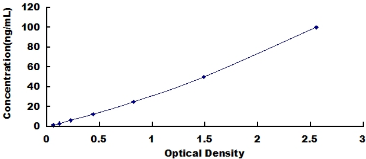
人抗肝素/血小板因子 4 抗体(Anti-HPF4)检测试剂盒标准曲线
