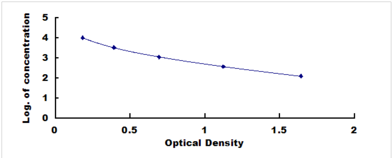
人绒毛膜促性腺激素 \alpha 肽 (CG \alpha ) 检测试剂盒标准曲线
