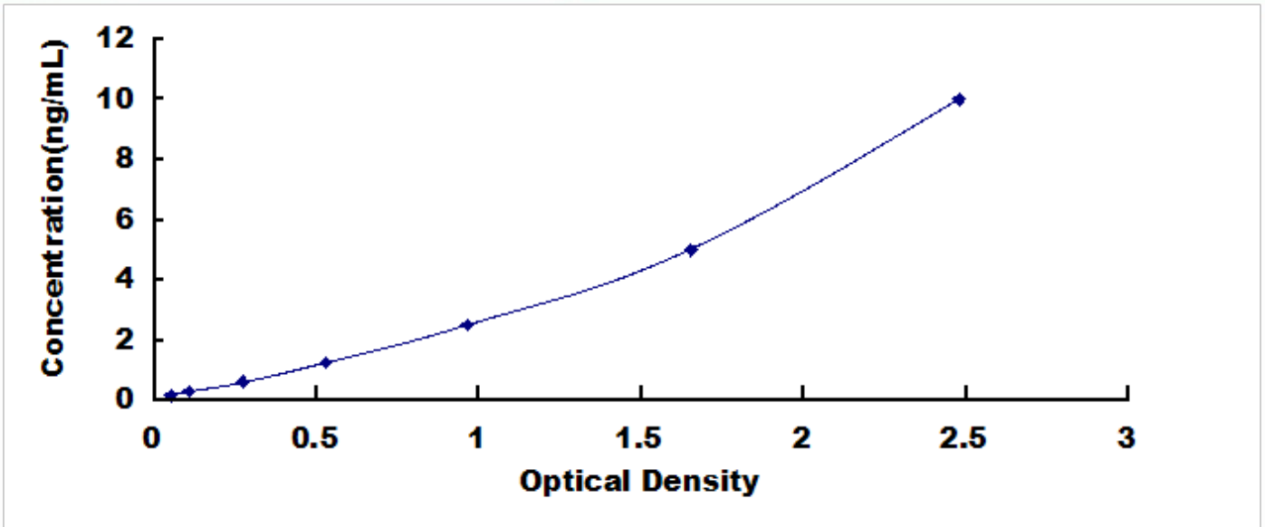
人生长关联蛋白 43 (GAP43) 检测试剂盒标准曲线
