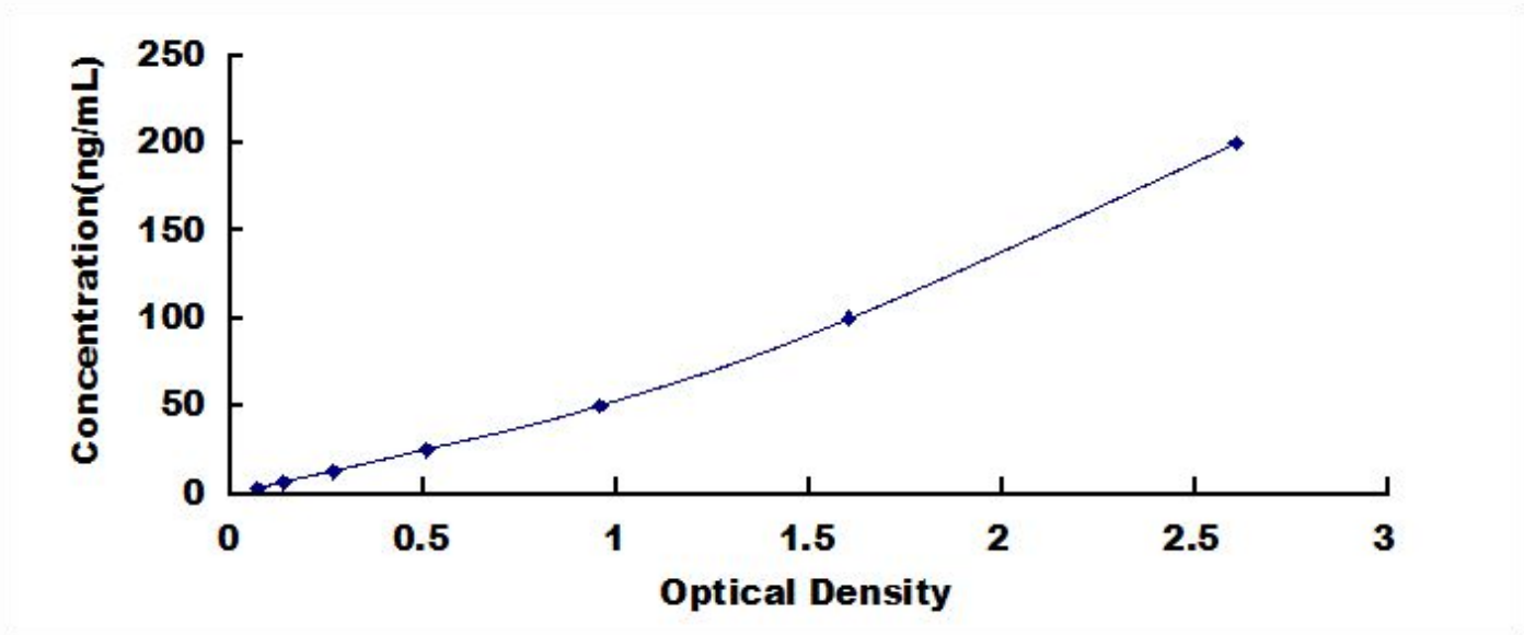
组蛋白 H2B (H2B) 检测试剂盒标准曲线
