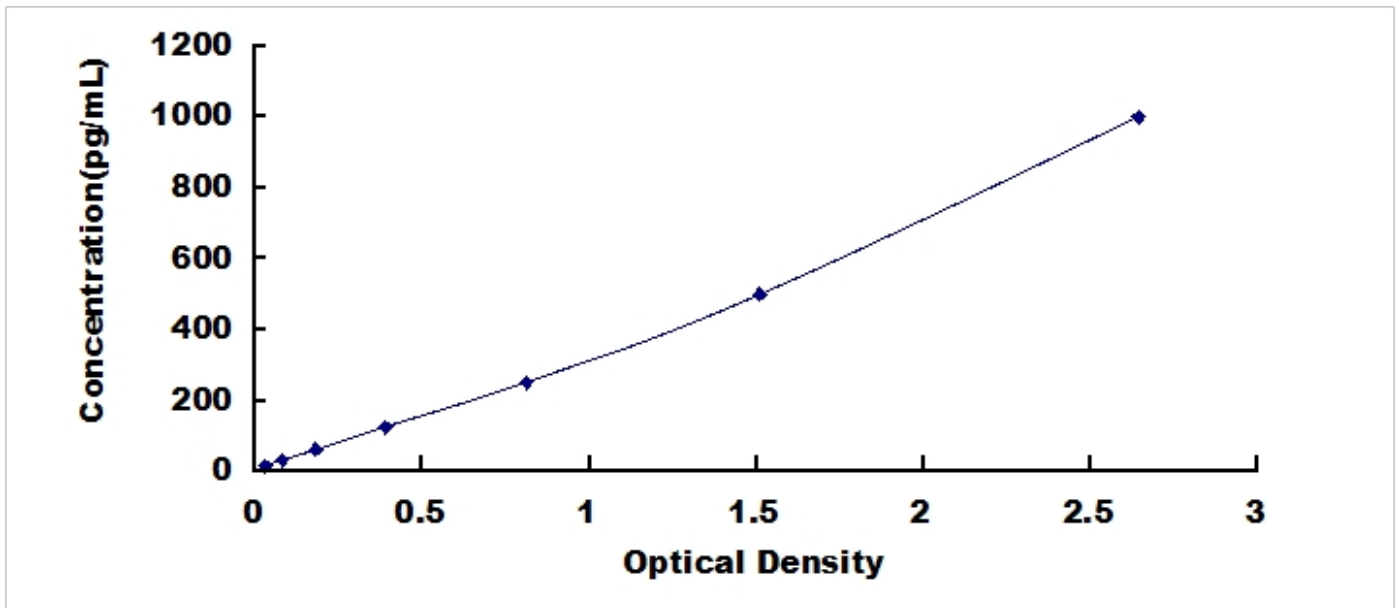
猪肿瘤坏死因子 \alpha (TNF \alpha ) 检测试剂盒标准曲线
