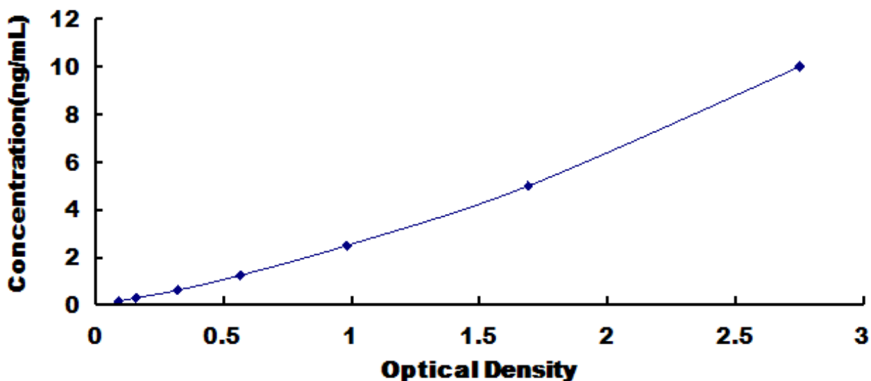
牛血清白蛋白(BSA)超敏检测试剂盒标准曲线
