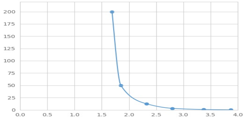
( I 型胶原交联氨基端肽)检测试剂盒标准曲线
