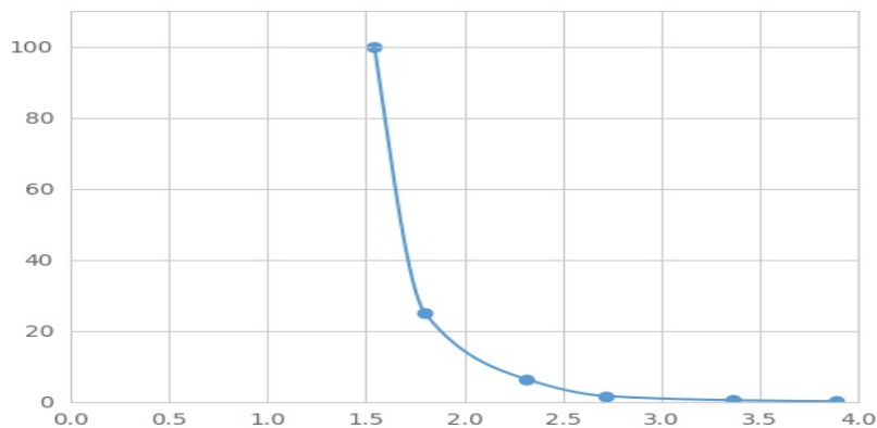
(肽聚糖) 检测试剂盒标准曲线
